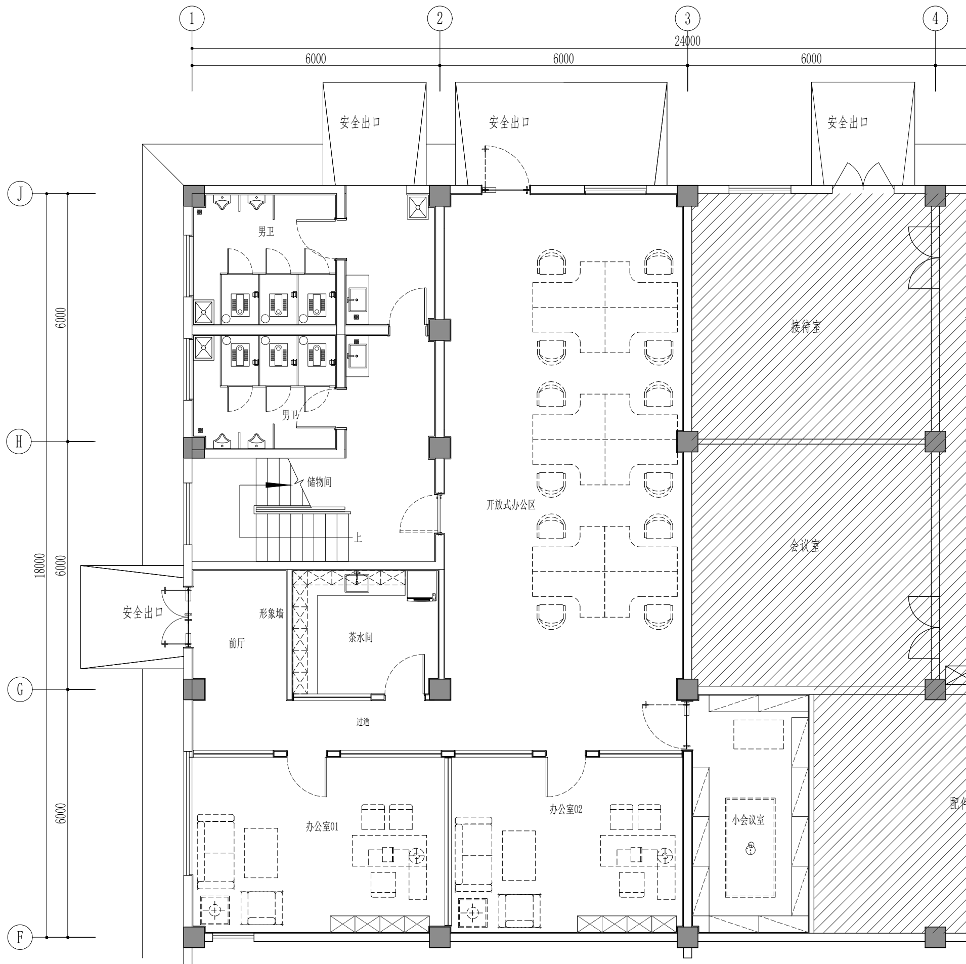
平面布置图 | 1:100
